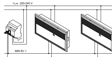
N.P. - No permanente con puesta en reposo. N.P. - Non maintained with standby. N.P. - Non permanent avec mise en veille.
