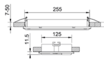
Empotrada en falso techo
