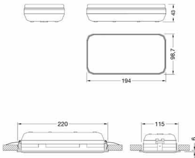
Empotrada en falso techo
