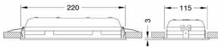
Empotrada en falso techo
